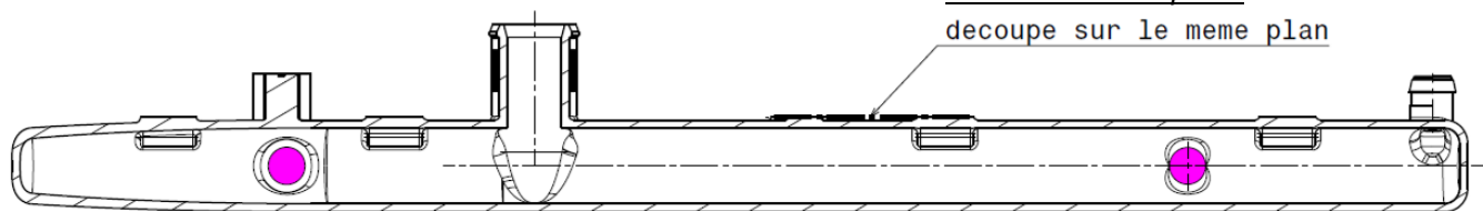
Coupe A-A
