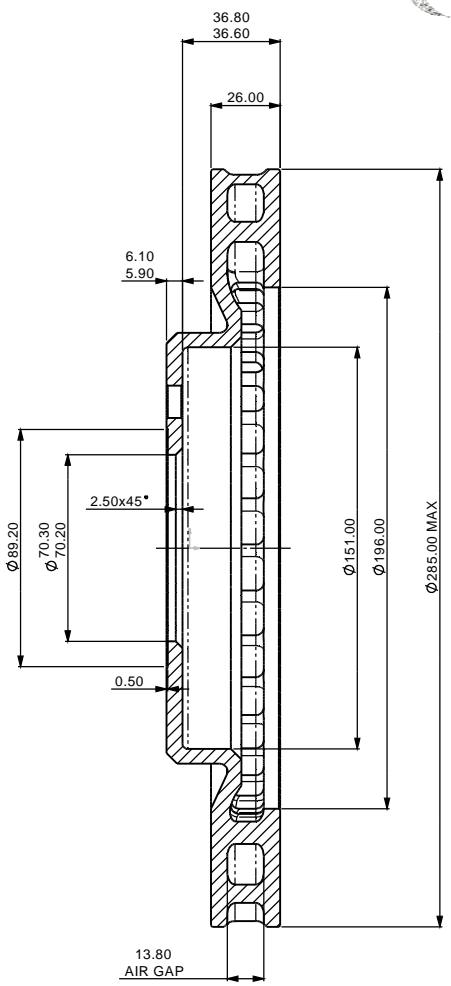
SECTION A-A
